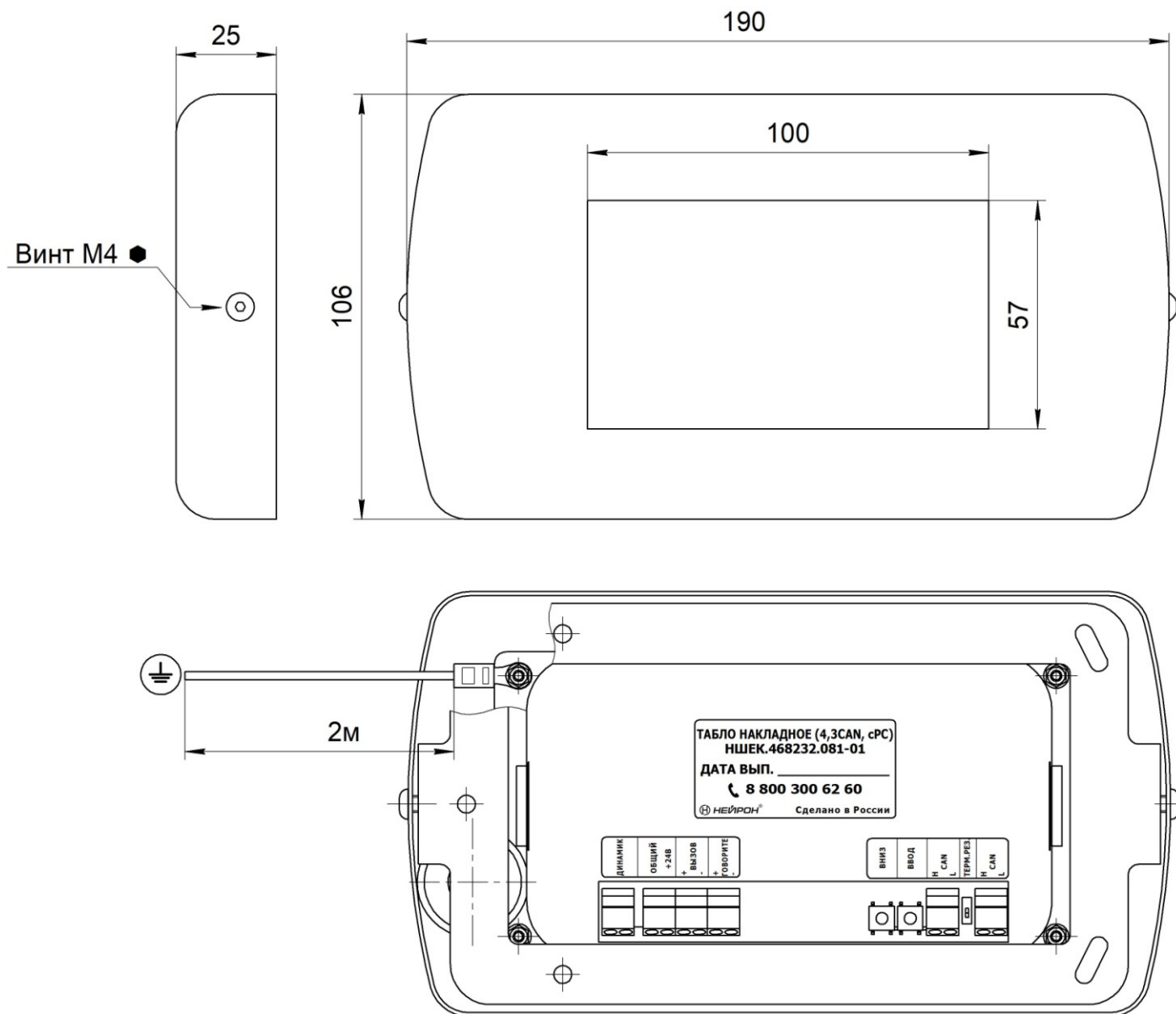
Рис.1 Внешний вид Табло накладное (4,3CAN, cPC) НШЕК.468232.081-01
